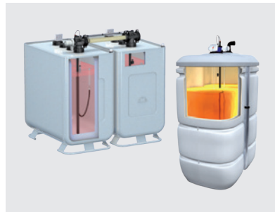
Moderne ein- und doppelwandige Sicherheitstanks Modern single and double-walled safety tanks
