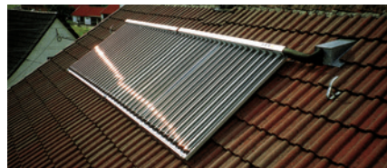
Anlagenbeispiel – Vakuumröhrenkollektor Example of solar installations – Vacuum tube collector
