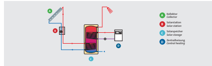
Standardsolaranlage zur Trinkwassererwärmung im Einfamilienhaus Standard solar thermal system for domestic hot water production in a detached house
